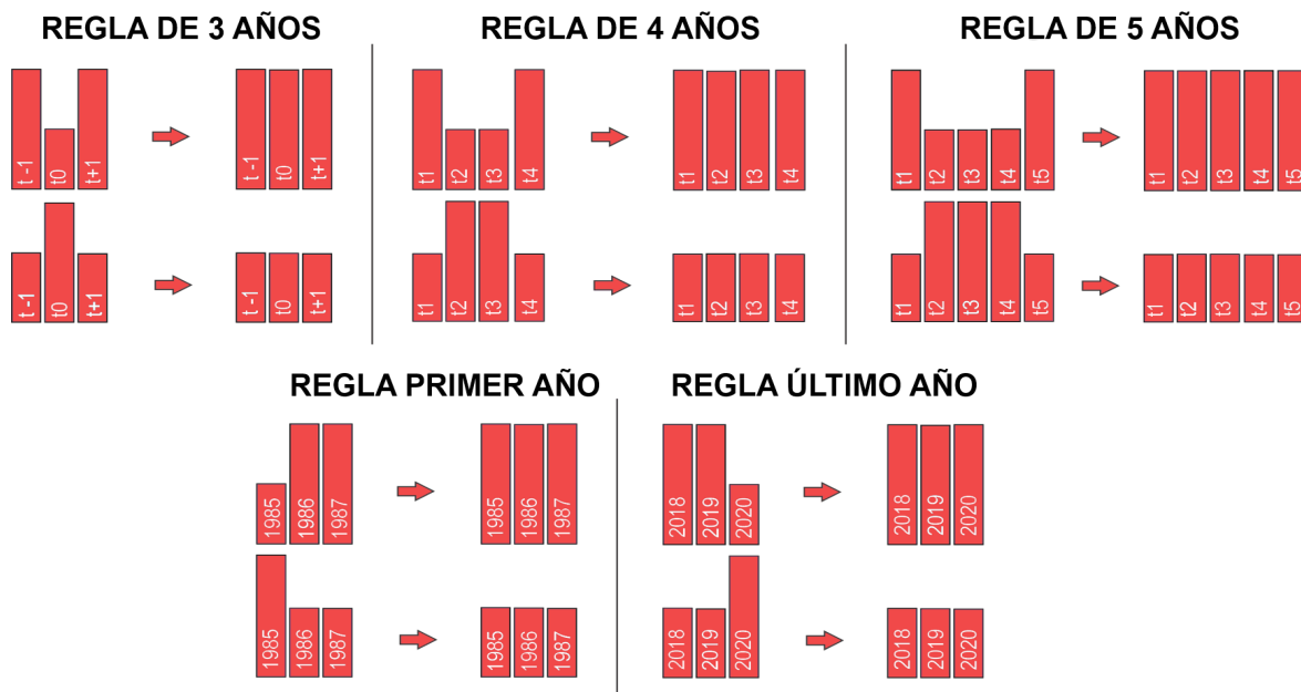
Figura 7. Filtro temporal.
