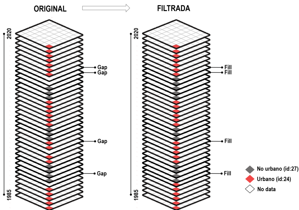
Figura 6. Filtro gapfill.
